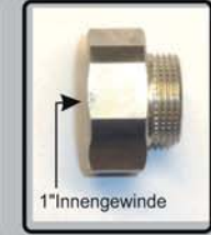
Best Nr: 97016 Reduzierung von 1" Eisenrohr auf 3/4" ( für 3/4"HK Ventil)
