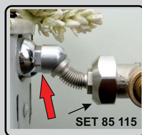
Winkel-Adapter für alle Superflex. Bild zeigt 3/4" HK- Ventilanschluß mit Set 85115
